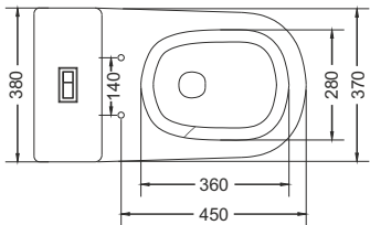
CASALE | S1013248 - S Trap 300 mm
