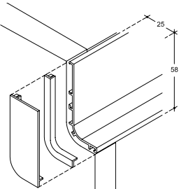
Passante fianco terminale anta base / Horizontal groove at end of side panel / Traversant porte module de base.
